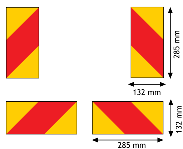
Obr. 2: Sada čtyř desek pro nákladní automobily
