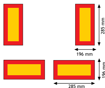
Obr. 2: Sada čtyř desek pro přívěsy a návěsy
